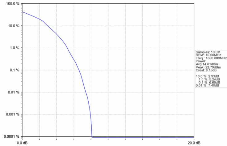
Band2_10MHz_16QAM_MCH_1880MHz_RB_27_0_NTNV
