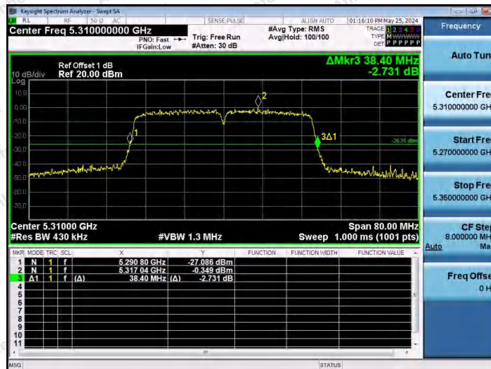
11N40SISO-Ant1-5310
