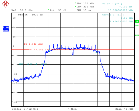
802.11n20_2462MHz 15.300MHz
