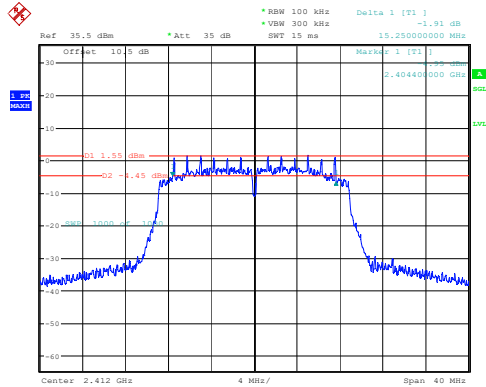
802.11n20_2412MHz 15.250MHz
