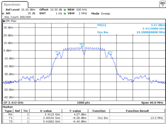
802.11b_2412MHz 13.200MHz
