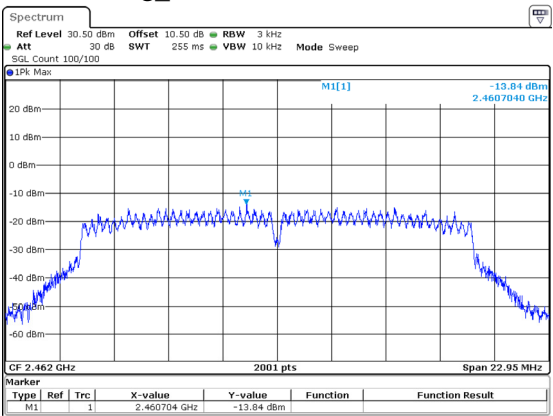
802.11g_2462MHz -13.84dBm/3kHz
