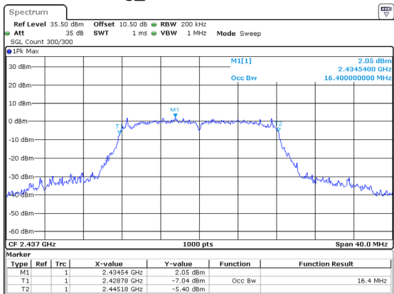
802.11g_2437MHz 16.400MHz
