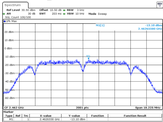
802.11b_2462MHz -13.10dBm/3kHz
