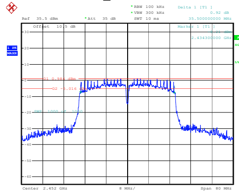
802.11n40_2452MHz 35.500MHz
