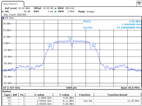
802.11b_2437MHz 13.160MHz
