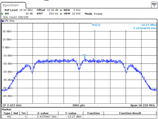
802.11b_2437MHz -13.27dBm/3kHz
