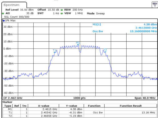
802.11b_2462MHz 13.160MHz
