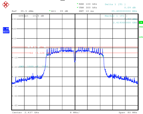
802.11n40_2437MHz 35.400MHz
