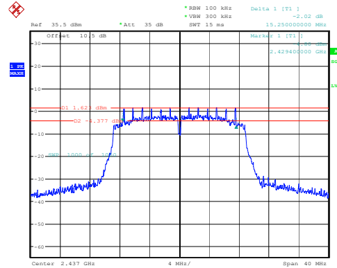
802.11n20_2437MHz 15.250MHz
