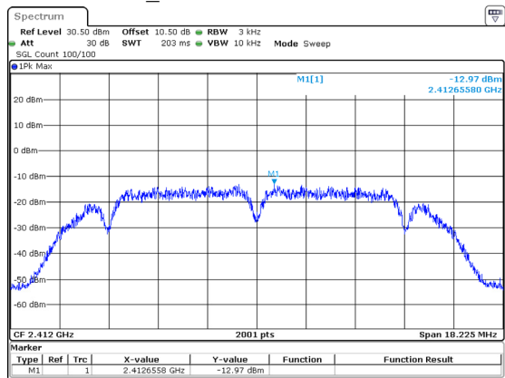
802.11b_2412MHz -12.97dBm/3kHz
