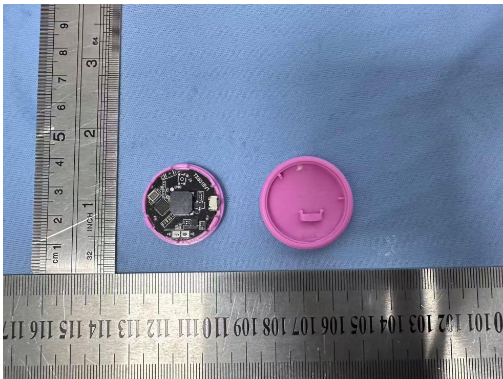
Internal Photos(TX03)
