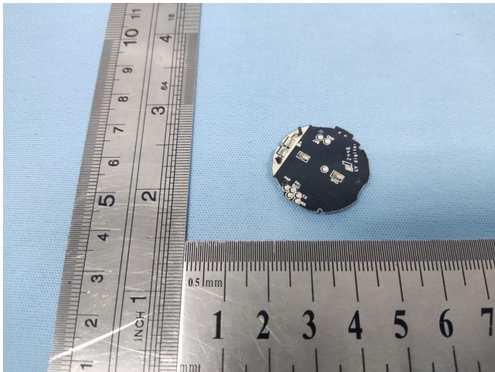
Internal Photos(TX02)
