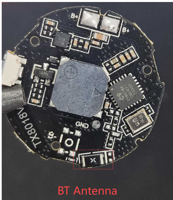
Internal Photos(TX02)
