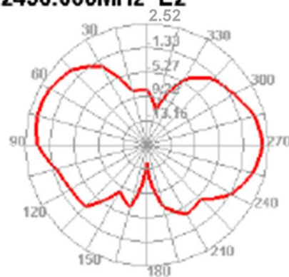
2450.000MHz E2
