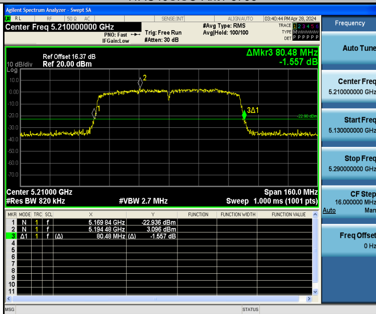
11AC80SISO-Ant1-5210
