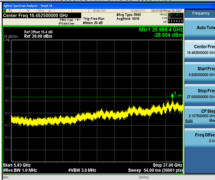
11AC80SISO-Ant1-5775-5925~27000-PASS
