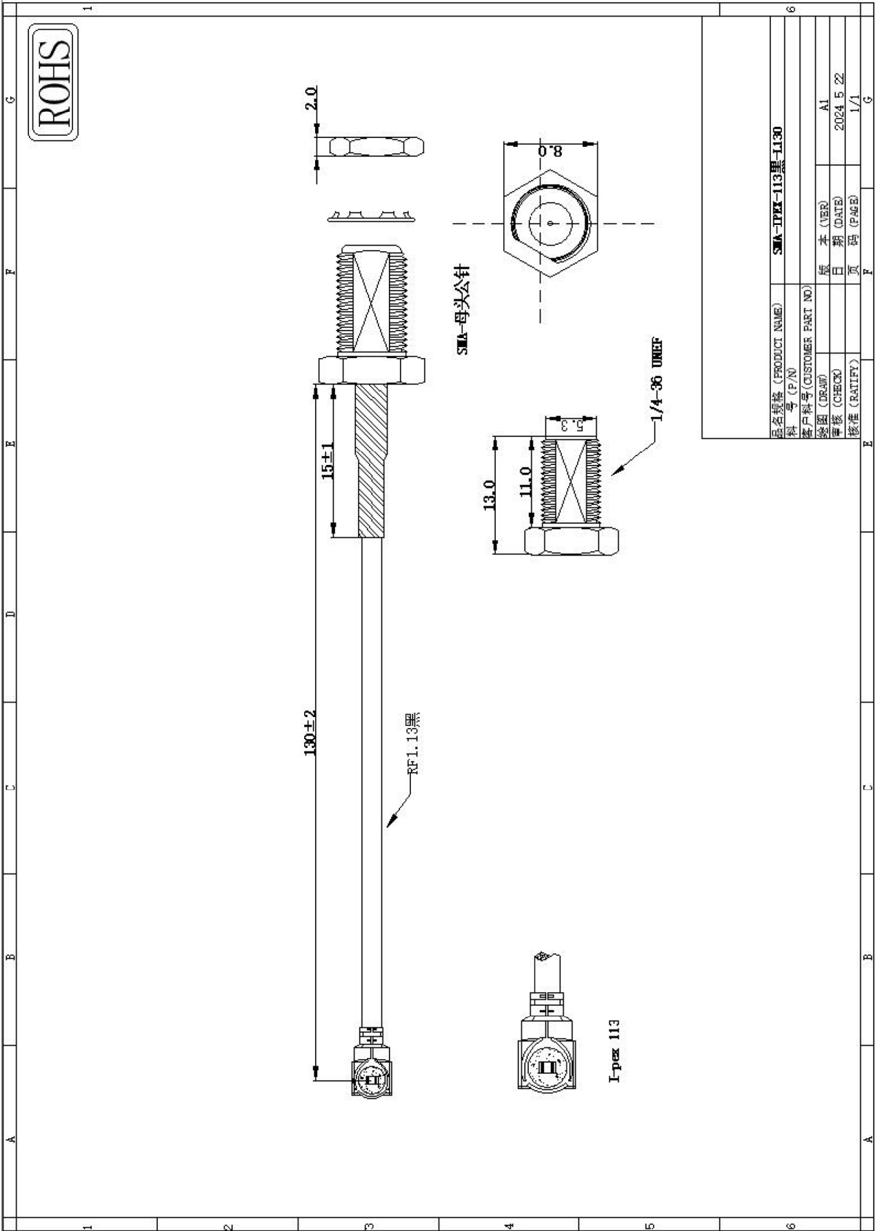
4.连接线结构图:
