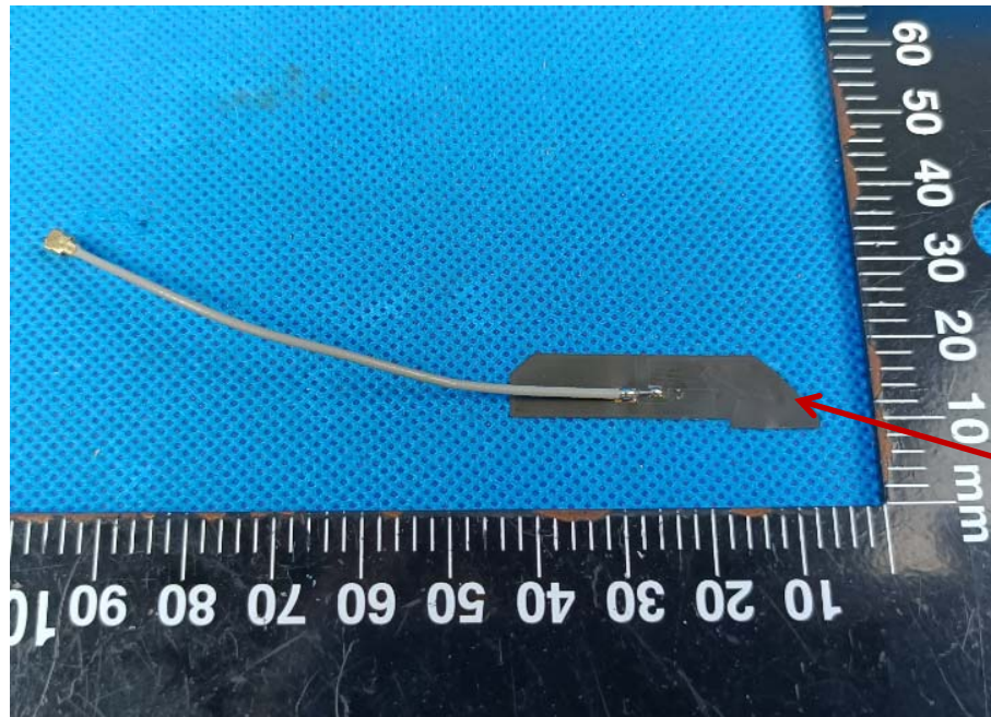
FPCB ANT
