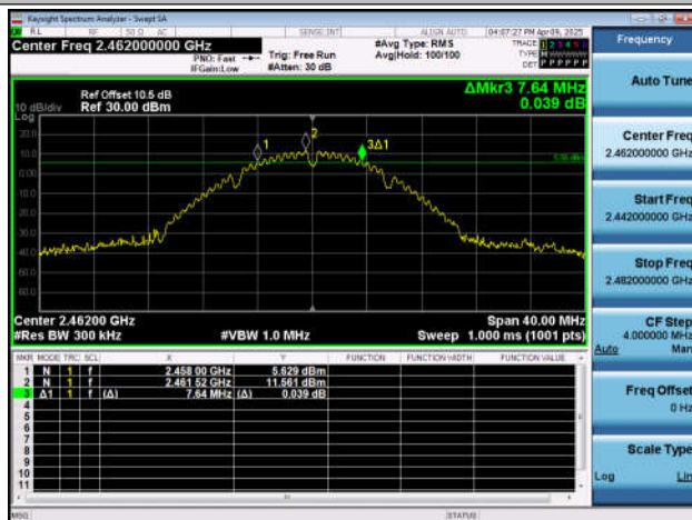
11B-Ant4-2462-PASS
