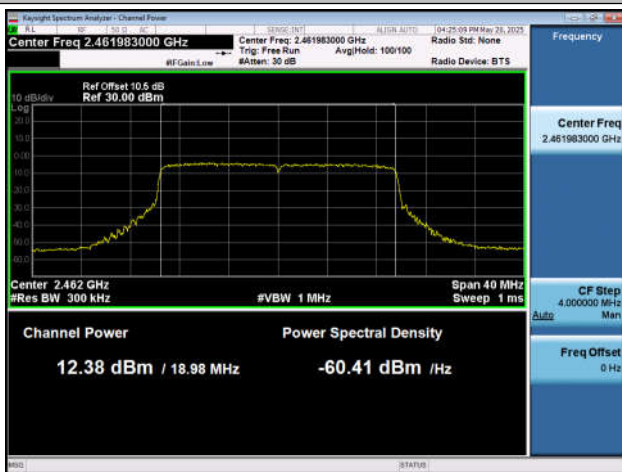
11AX20MIMO-Ant4-2462-PASS
