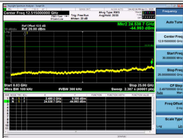
BLE 2M-Ant4-2480-30~25000-PASS
