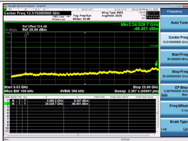
BLE 2M-Ant7-2480-30~25000-PASS
