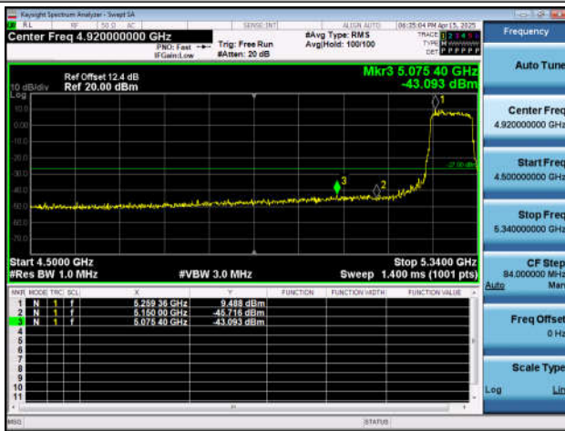
11AX80SISO-Ant6-5290-PASS
