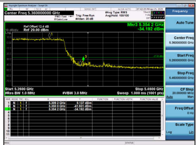
11BE80SISO-Ant4-5290-PASS
