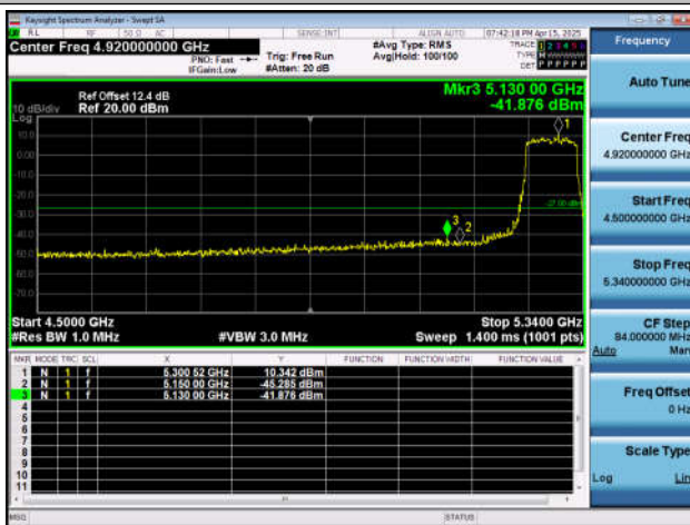
11BE80SISO-Ant4-5290-PASS
