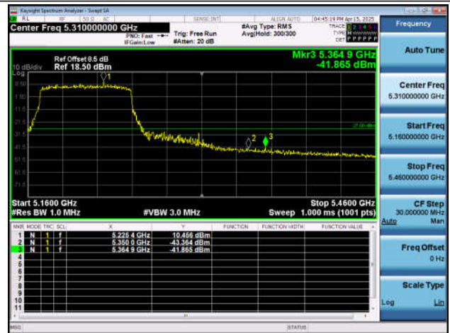
11BE80SISO-Ant4-5210-PASS
