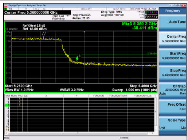
11AX80SISO-Ant6-5290-PASS
