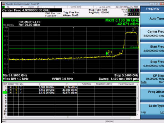
11AC80SISO-Ant6-5290-PASS
