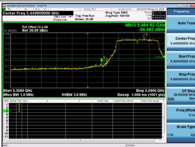
11AC80SISO-Ant4-5530-PASS
