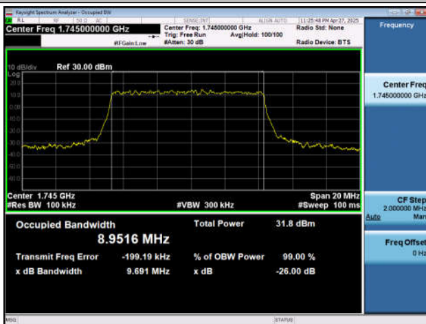
NTNV-n66-PC3-15-10-M-DFT-QPSK-Outet_Full-Ant1-PAS
