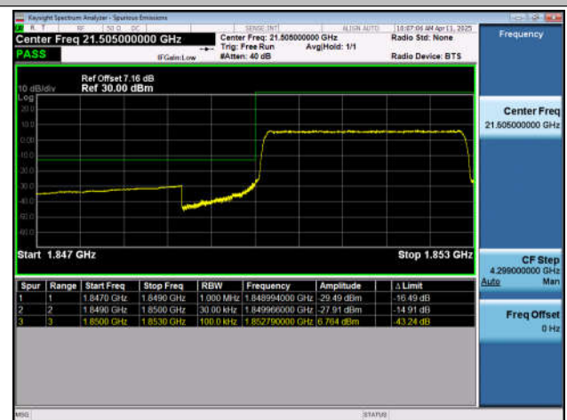
Band2-3MHz-QPSK-18615-15RB#0-PASS
