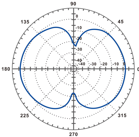
垂直 Pattern
