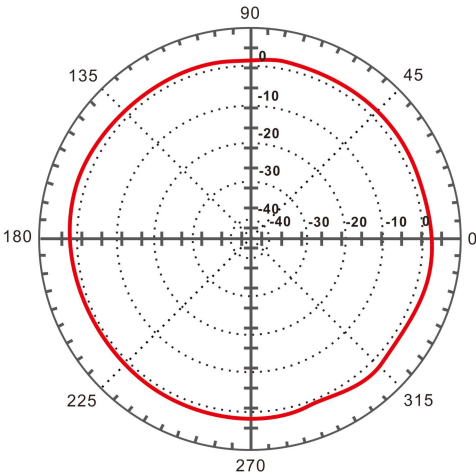
水平 Pattern
