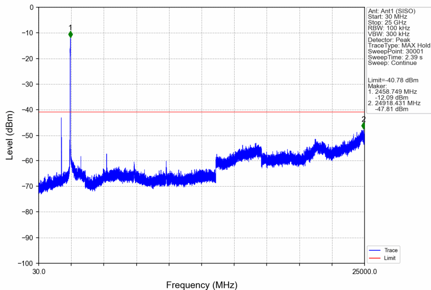
802.11n(HT40)_HCH_2452MHz_Ant1 (SISO)_NTNV
