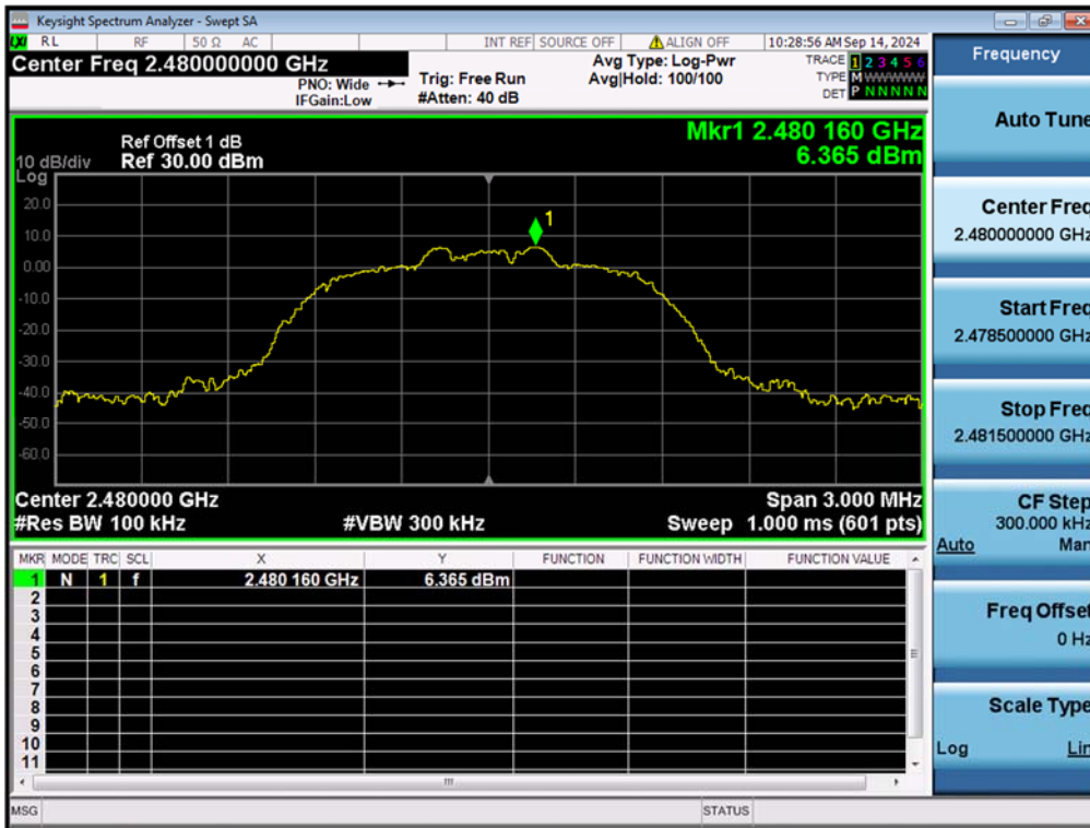
Band Edge
