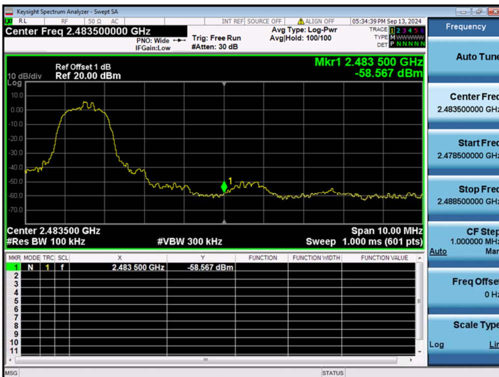
Band Edge
