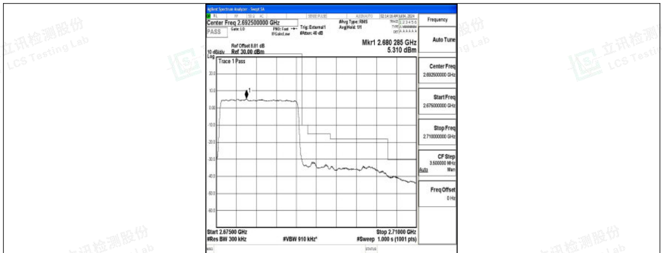
Band41_15MHz_QPSK_41515_75RB#0
