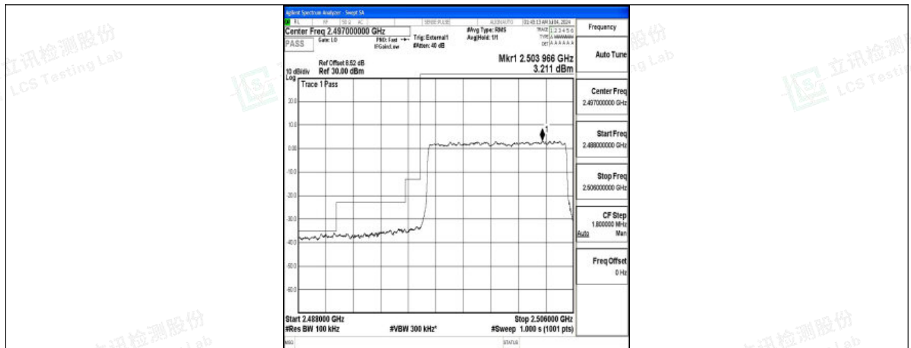
Band41_10MHz_QPSK_39700_50RB#0
