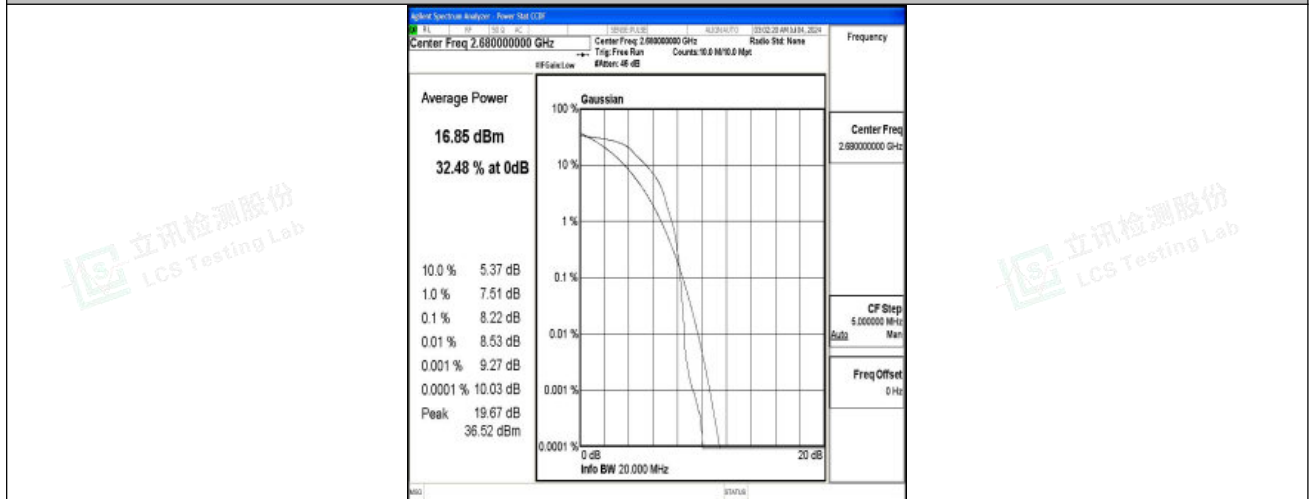
Band41-20MHz-QPSK-41490-1RB#0-PASS
