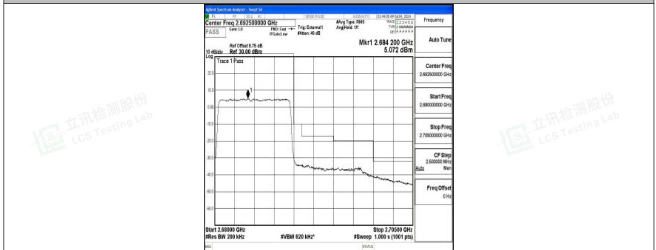
Band41_10MHz_QPSK_41540_50RB#0
