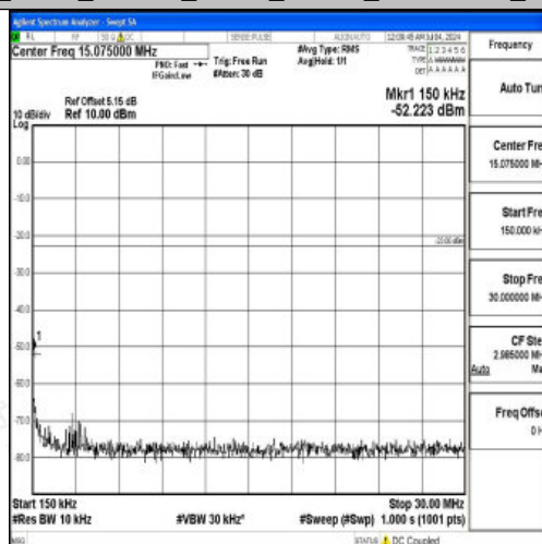
Band26 5MHz 16QAM 26915 1RB#0 0.15~30 0.15~30
