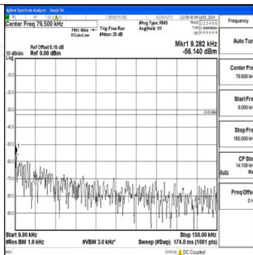
Band26 5MHz 16QAM 26915 1RB#0 0.009~0.15 0.009~0.15
