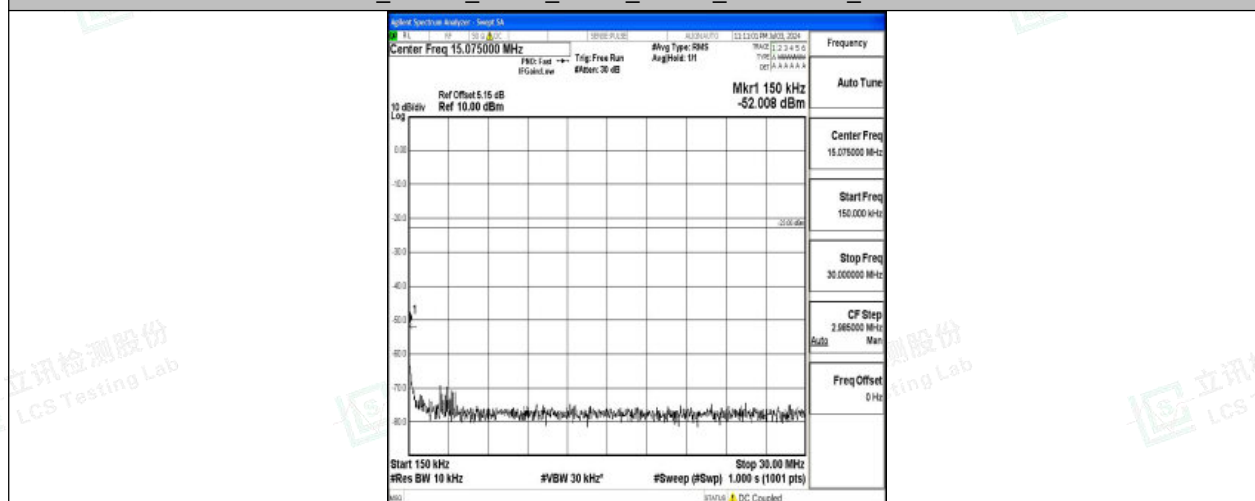
Band26 10MHz QPSK 26740 1RB#0 0.15~30 0.15~30
