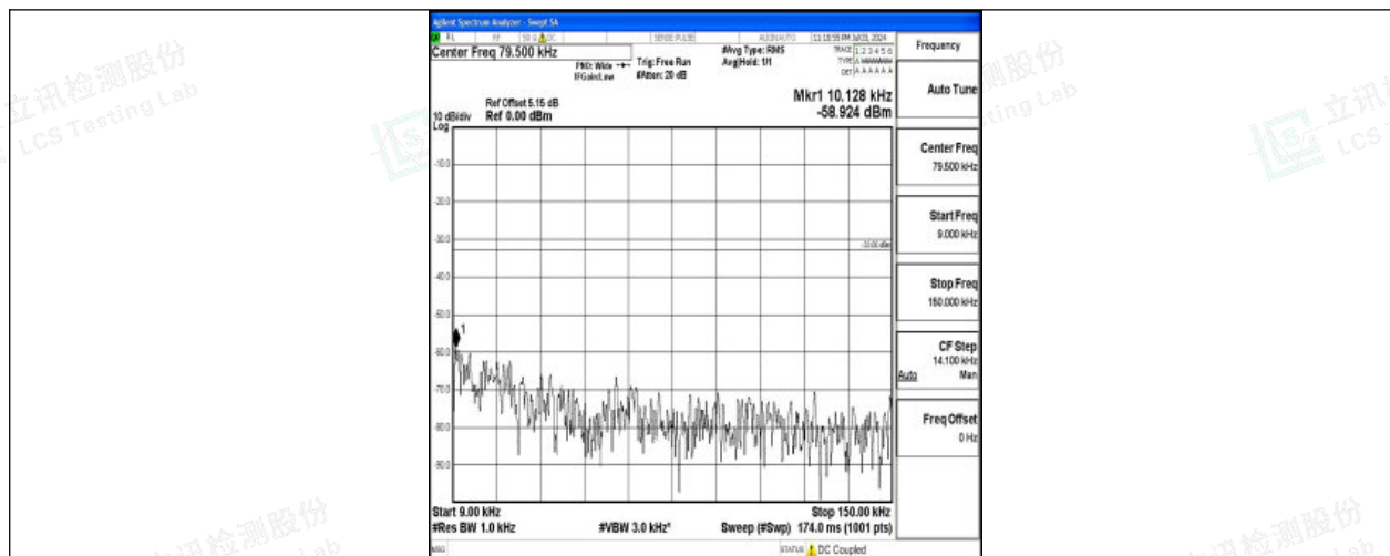
Band26 10MHz QPSK 26740 1RB#0 0.009~0.15 0.009~0.15
