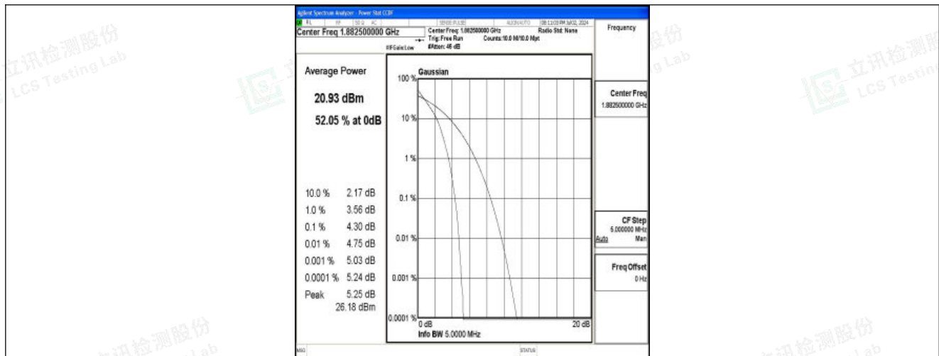
Band25-3MHz-QPSK-26365-15RB#0-PASS
