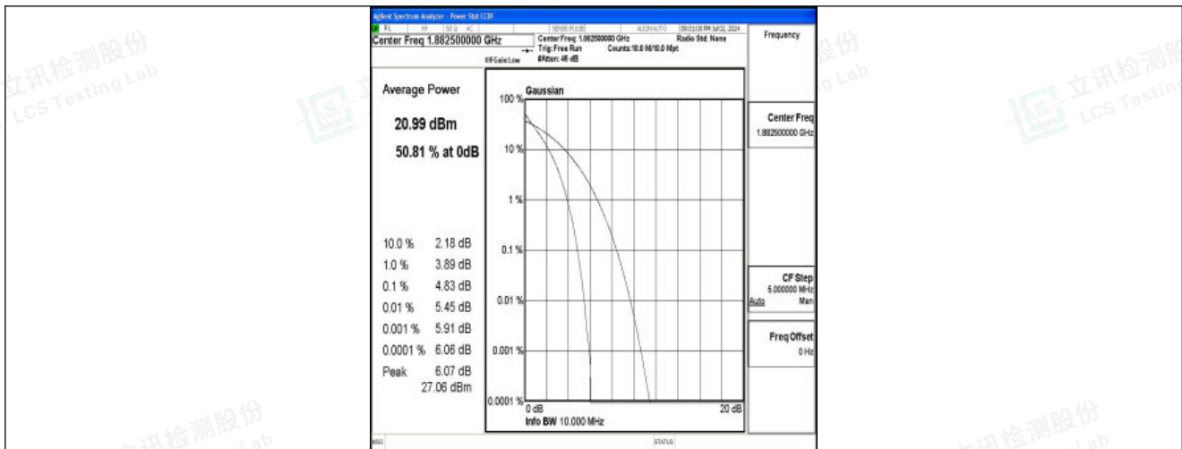
Band25-10MHz-QPSK-26365-50RB#0-PASS
