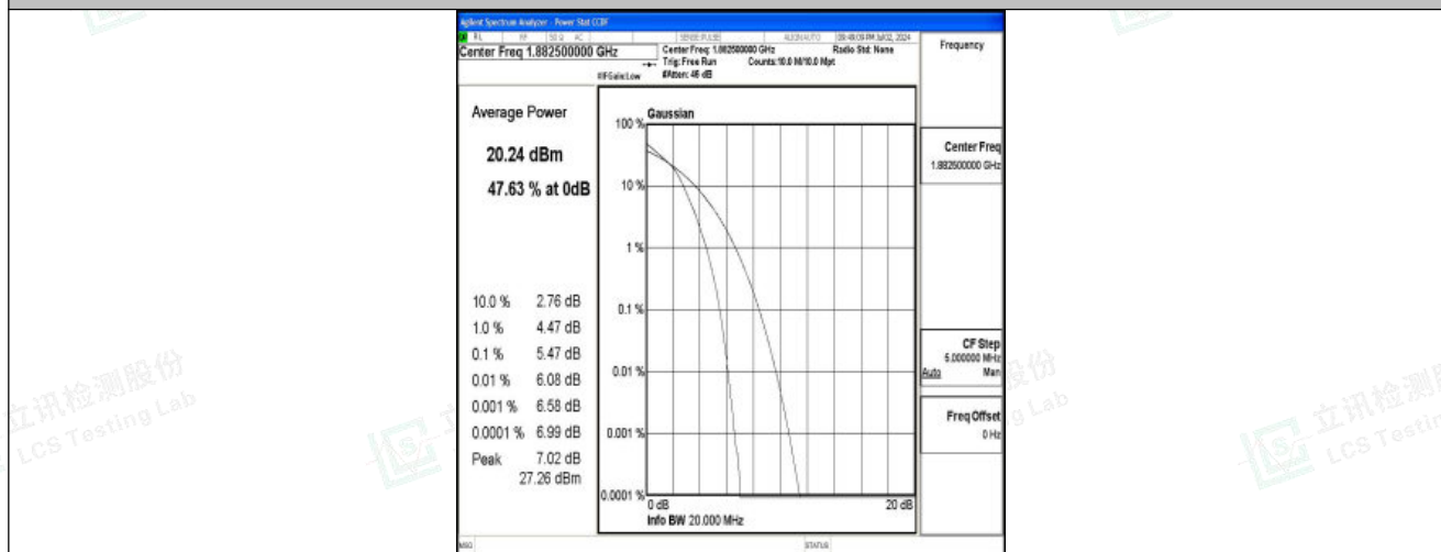
Band25-20MHz-16QAM-26365-100RB#0-PASS
