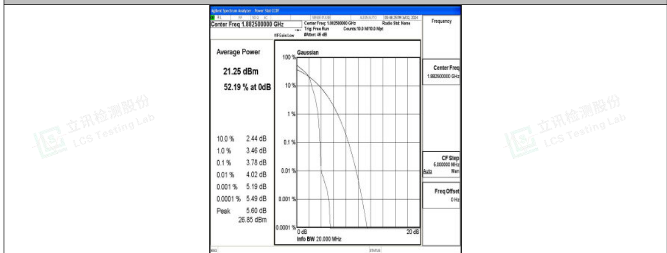
Band25-20MHz-16QAM-26365-1RB#0-PASS
