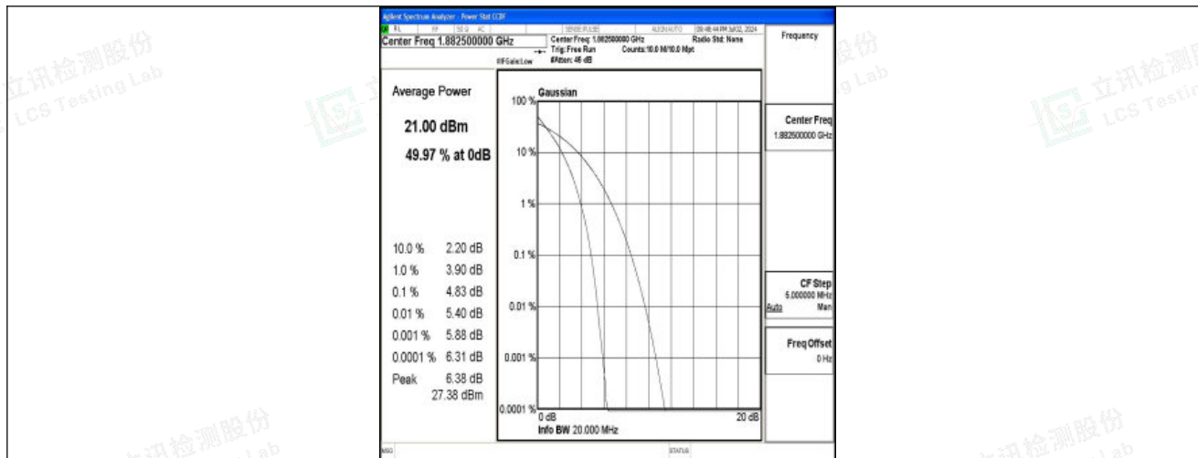
Band25-20MHz-QPSK-26365-100RB#0-PASS
