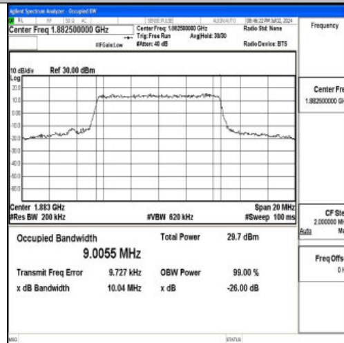
Band25-10MHz-QPSK-26365-50RB#0-PASS
