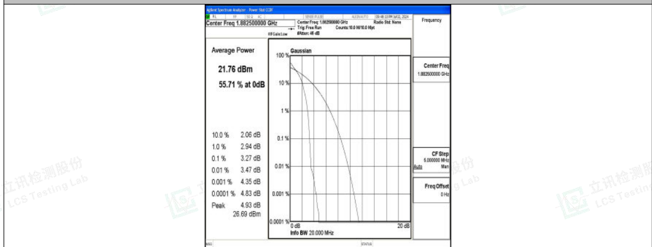
Band25-20MHz-QPSK-26365-1RB#0-PASS
