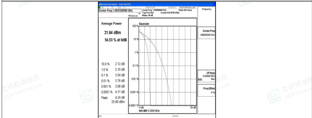
Band25-5MHz-QPSK-26365-1RB#0-PASS
