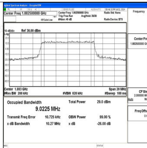
Band25-10MHz-16QAM-26365-50RB#0-PASS
