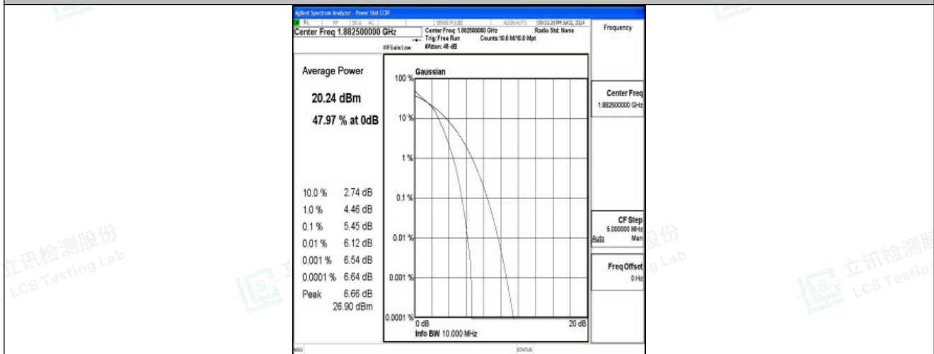
Band25-10MHz-16QAM-26365-50RB#0-PASS
