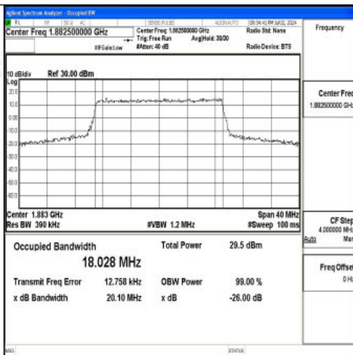
Band25-20MHz-16QAM-26365-100RB#0-PASS
