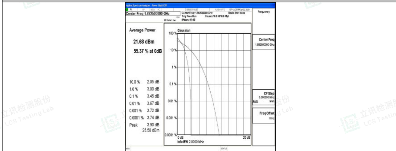
Band25-1.4MHz-QPSK-26365-1RB#0-PASS
