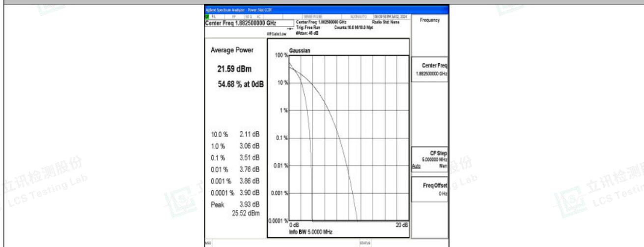
Band25-3MHz-QPSK-26365-1RB#0-PASS
