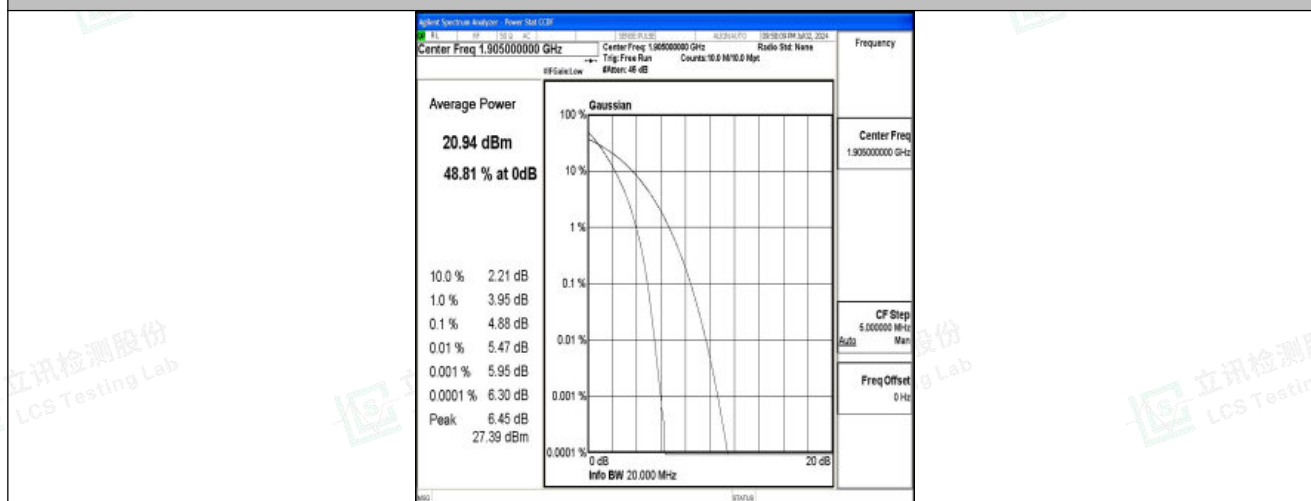
Band25-20MHz-QPSK-26590-100RB#0-PASS
