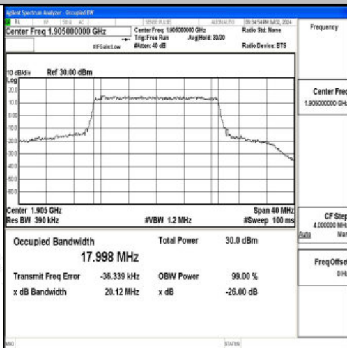
Band25-20MHz-QPSK-26590-100RB#0-PASS
