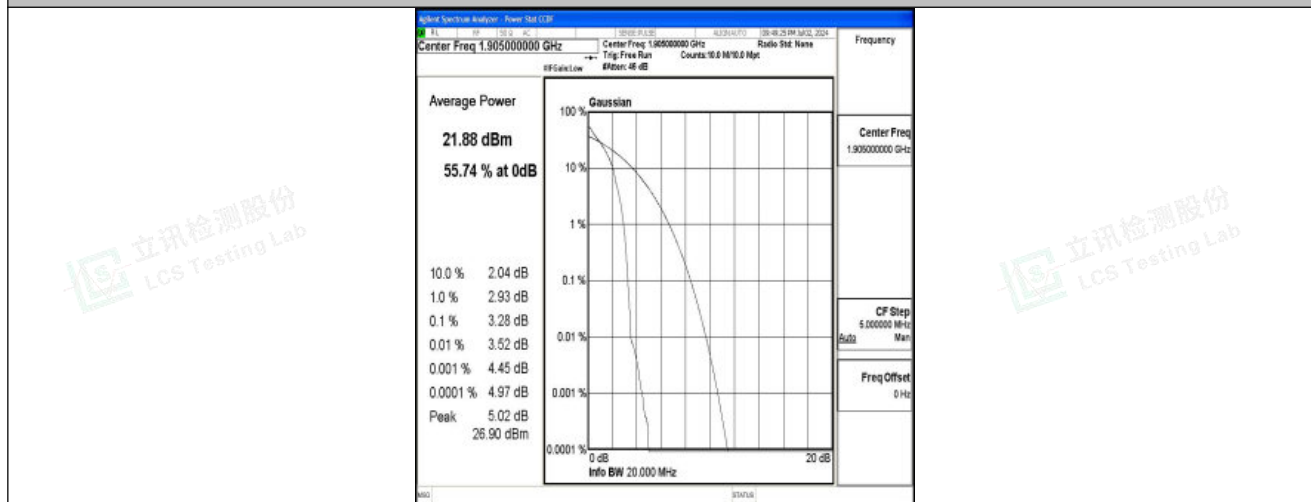
Band25-20MHz-QPSK-26590-1RB#0-PASS
