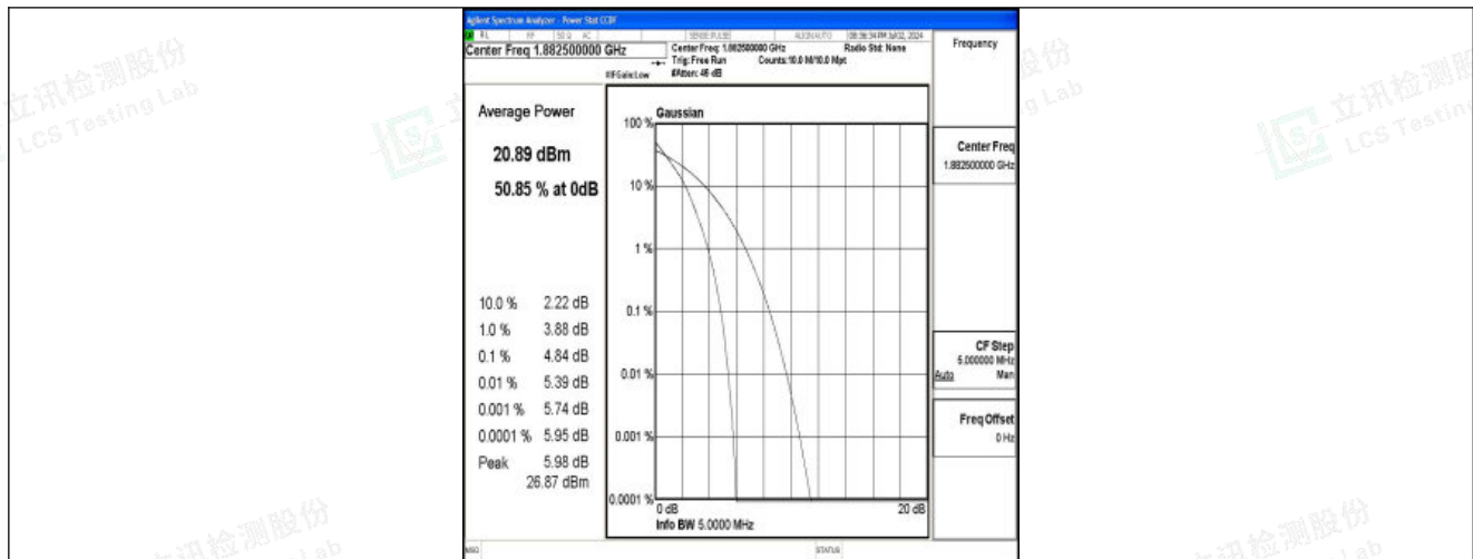
Band25-5MHz-QPSK-26365-25RB#0-PASS
