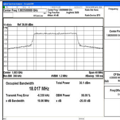
Band25-20MHz-QPSK-26365-100RB#0-PASS
