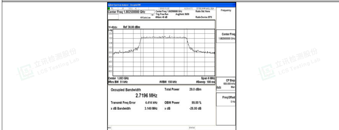
Band25-3MHz-QPSK-26365-15RB#0-PASS
