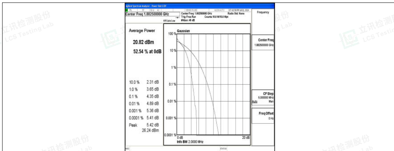
Band25-1.4MHz-QPSK-26365-6RB#0-PASS
