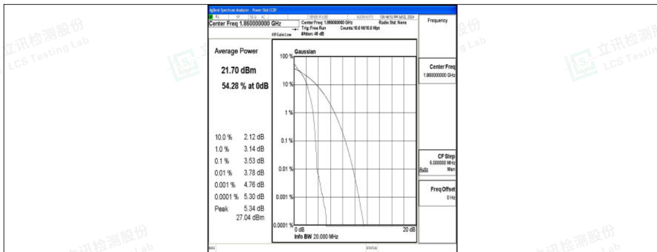
Band25-20MHz-QPSK-26140-1RB#0-PASS
