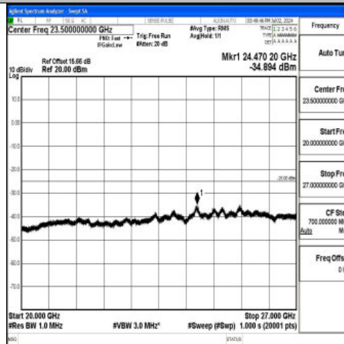
Band7_20MHz_QPSK_20850_1RB#0_20000~27000_20000~27000
