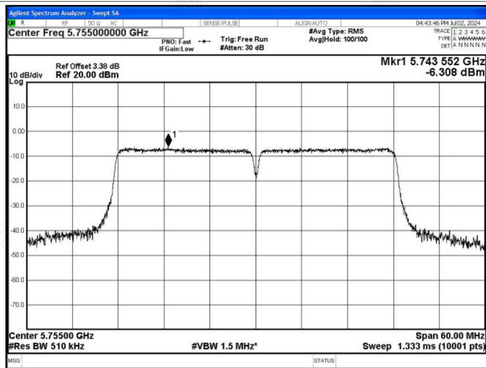
PSD HVHT ac40 5755MHz Ant1
