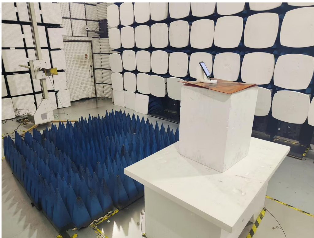
Fig. 3 (Above 1 GHz)
