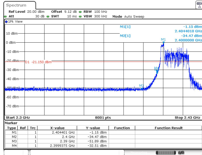
11AX20SISO_Ant1_Low_2412_26Tone_RU0
