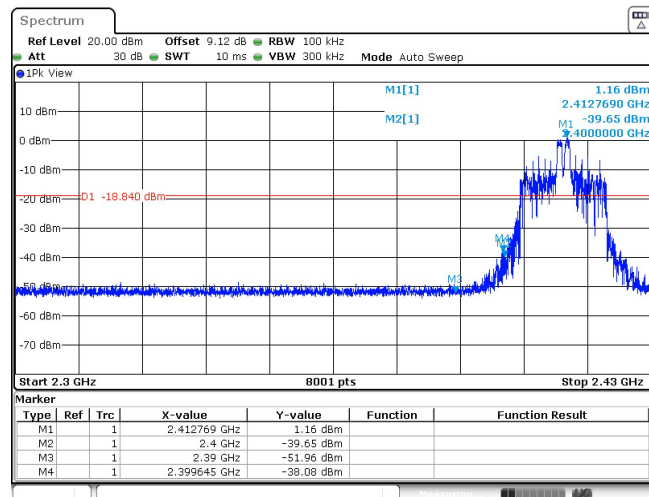
11AX20SISO_Ant1_Low_2412_26Tone_RU0
