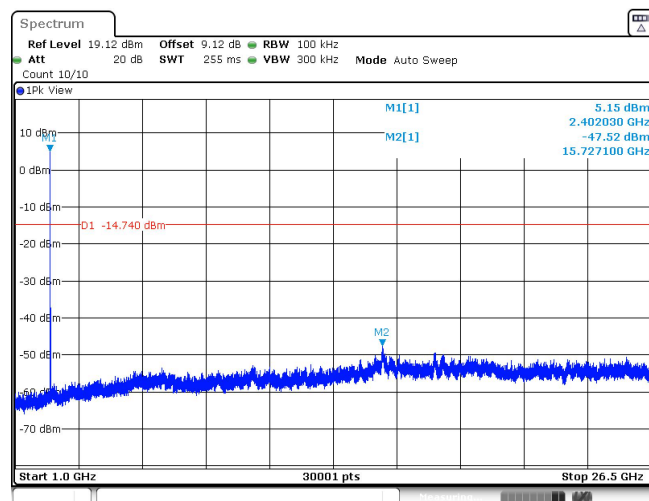
BLE_2M_Ant1_2402_1000~26500
