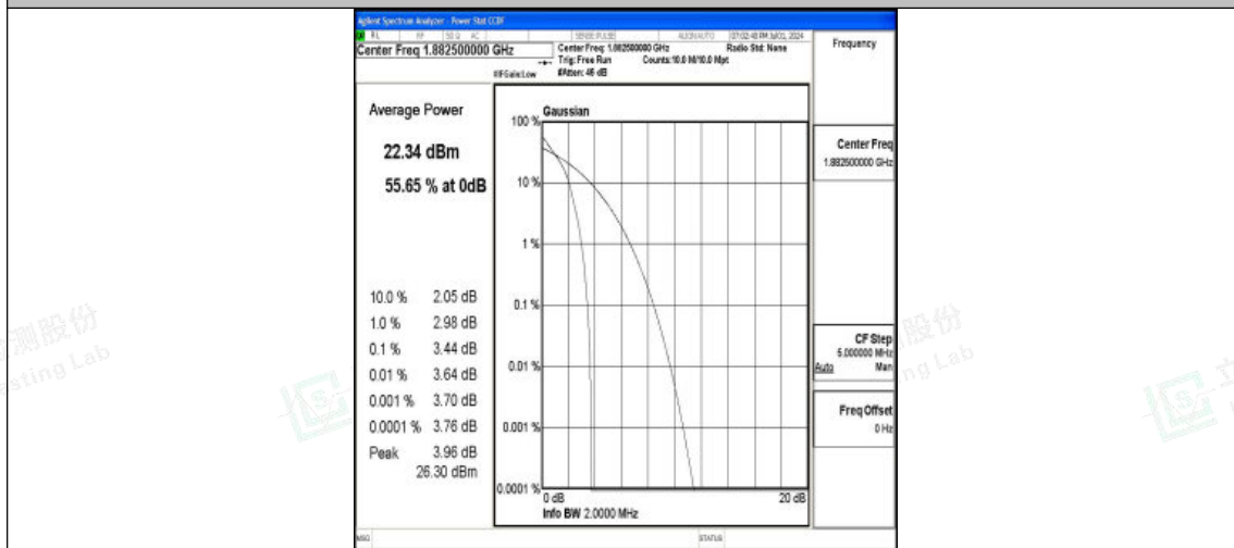
Band25-1.4MHz-QPSK-26365-1RB#0-PASS
