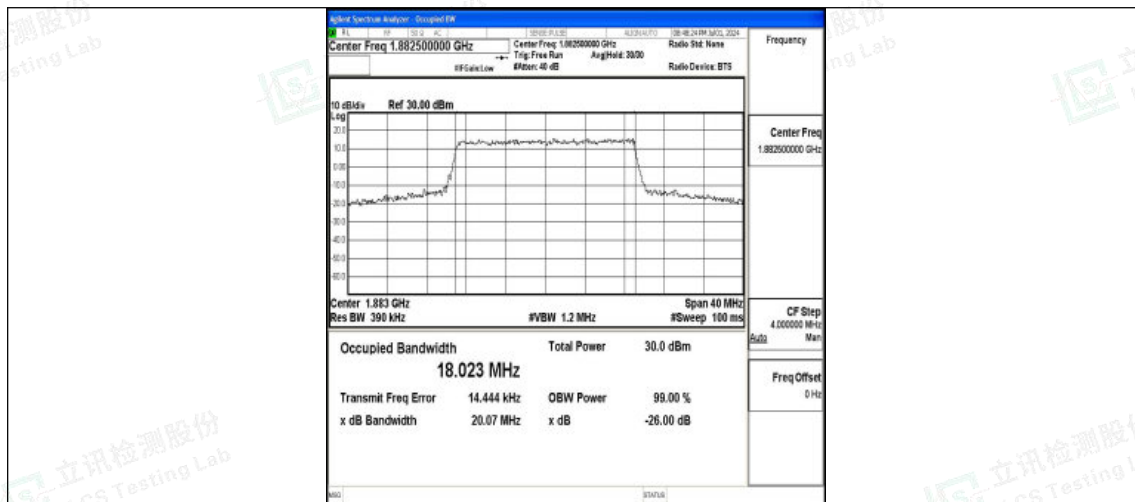
Band25-20MHz-16QAM-26365-100RB#0-PASS
