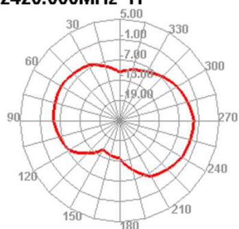
2420.000MHz H
