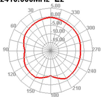
2410.000MHz E2
