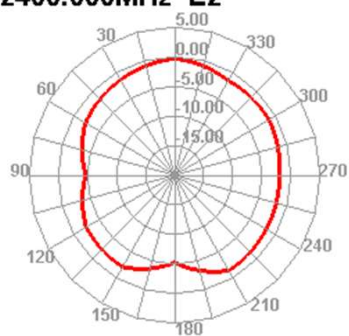
2400.000MHz E2
