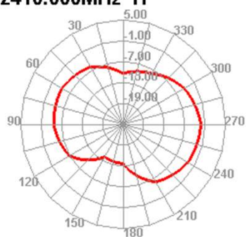
2410.000MHz H
