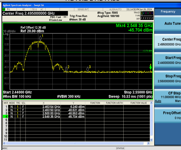
11B-Ant2-2462-PASS
