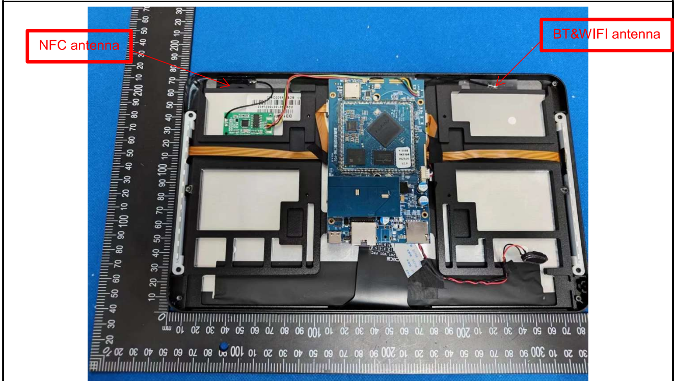
EUT Photo
