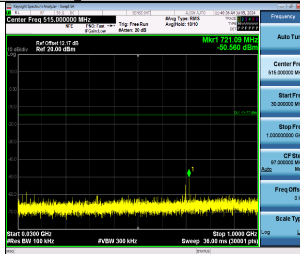
BLE 1M-Ant1-2402-30~1000-PASS
