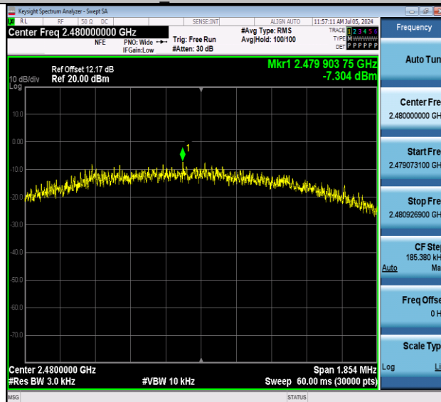
BLE 2M-Ant1-2480-PASS
