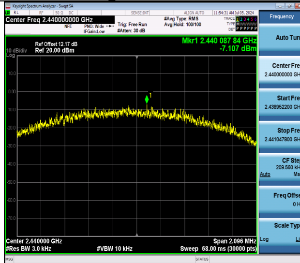
BLE 2M-Ant1-2440-PASS
