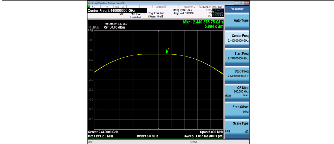
BLE 2M-Ant1-2440-PASS
