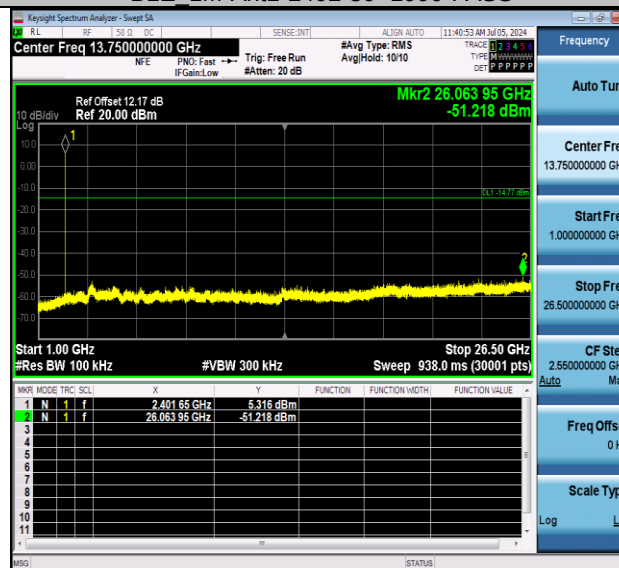
BLE 1M-Ant1-2402-1000~26500-PASS
