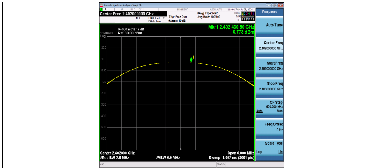
BLE 2M-Ant1-2402-PASS
