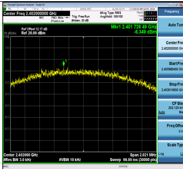
BLE 2M-Ant1-2402-PASS
