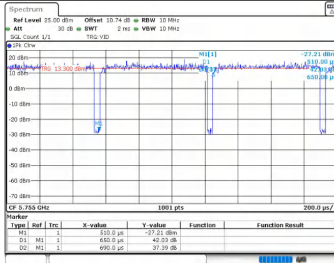
11N40MIMO_Ant2_5755
