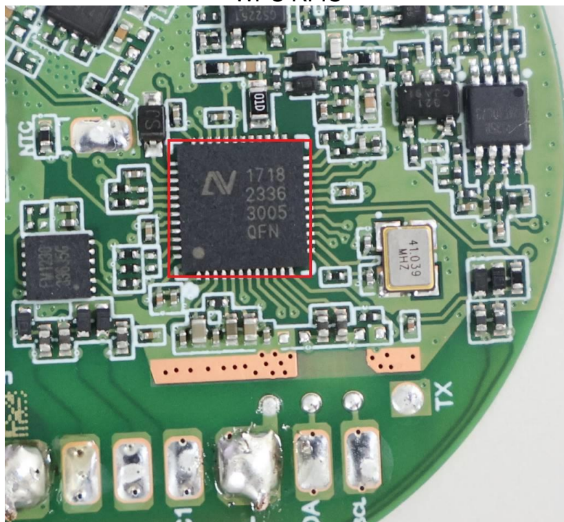
WPC RFIC
