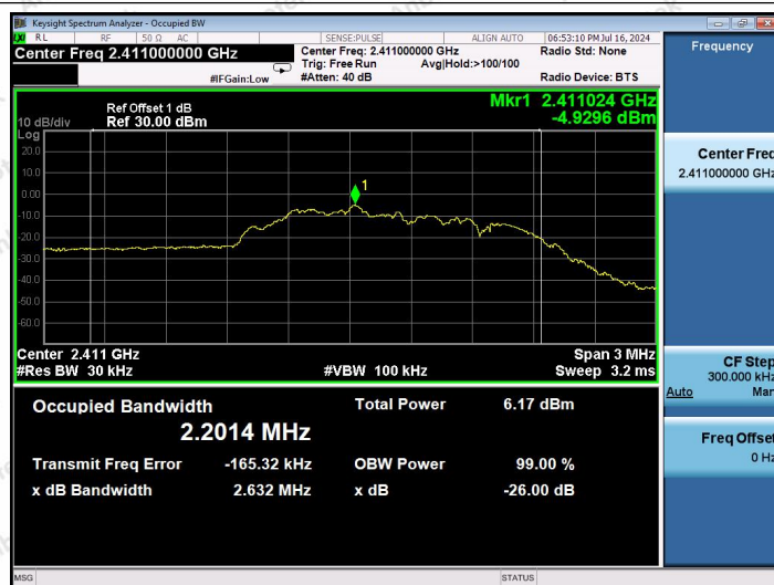
2.4G-Ant1-2411
