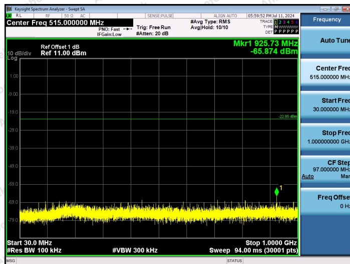
2.4G-Ant1-2411-30~1000-PASS
