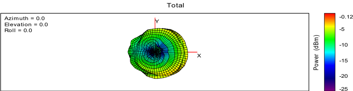
2360MHz TRP 1
