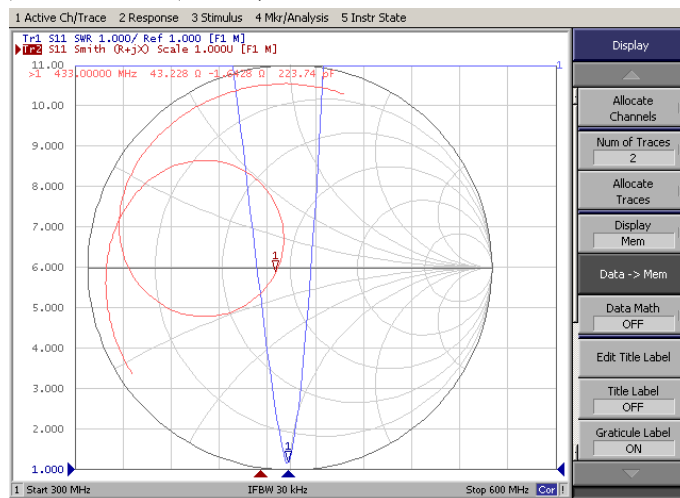
S11 ( VSWR 、 Return loss 、 Smith) Data
