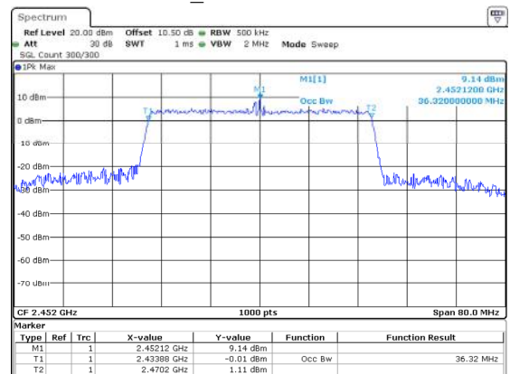
802.11n40_2452MHz 36.320MHz
