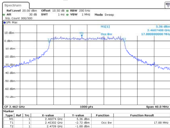
802.11n20_2462MHz 17.880MHz
