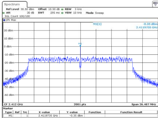
802.11n20_2412MHz -0.35dBm/3kHz
