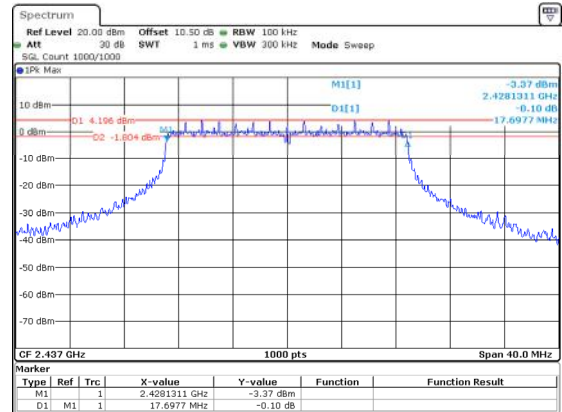
802.11n20_2437MHz 17.698MHz
