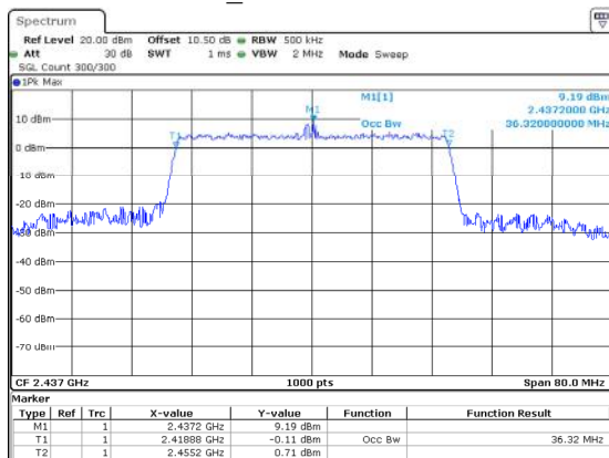
802.11n40_2437MHz 36.320MHz
