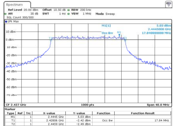
802.11n20_2437MHz 17.840MHz
