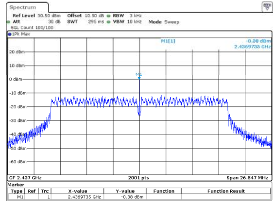
802.11n20_2437MHz -0.38dBm/3kHz
