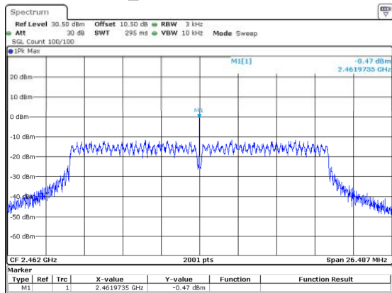
802.11n20_2462MHz -0.47dBm/3kHz
