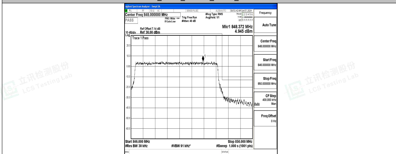
Band5_3MHz_QPSK_20635_15RB#0
