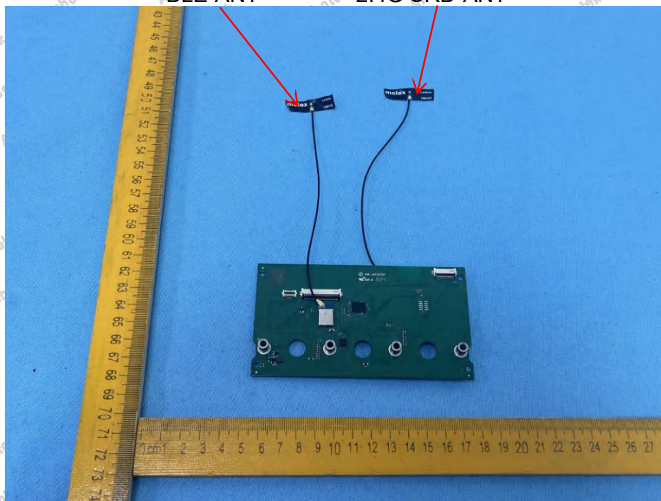
BLE-ANT
