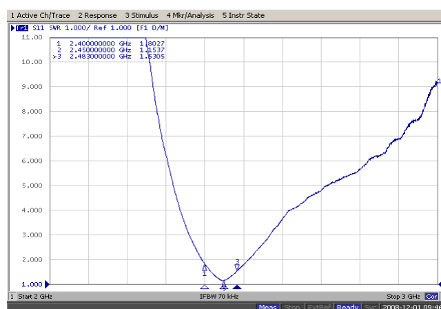
VSWR(S 11 )
