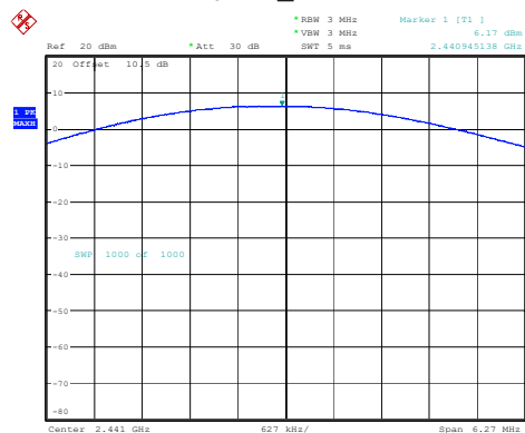
\pi/4 -DQPSK_Middle 6.17dBm
