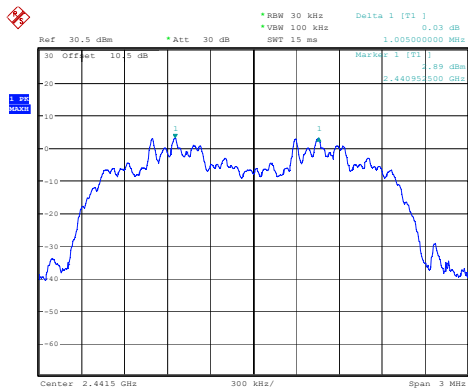
\pi/4 -DQPSK_Middle 1.005MHz
