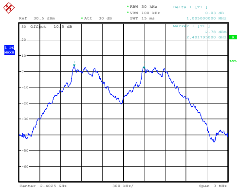
GFSK_Low 1.005MHz
