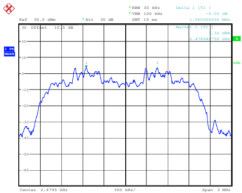
\pi/4 -DQPSK_High 1.005MHz
