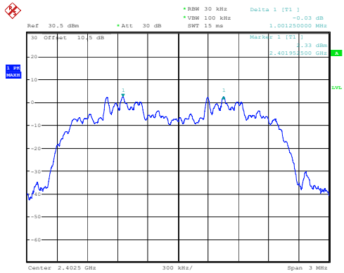
\pi/4 -DQPSK_Low 1.001MHz
