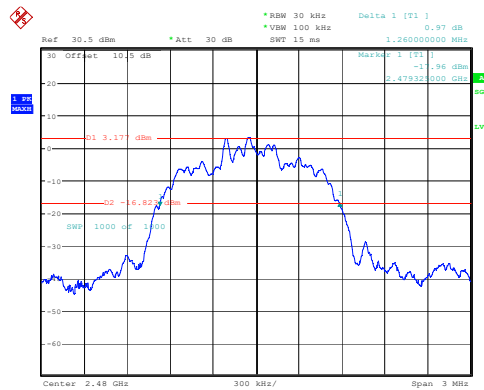
\pi/4 -DQPSK_High 1.260MHz
