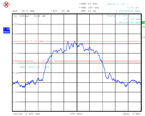
\pi/4 -DQPSK_Low 1.253MHz
