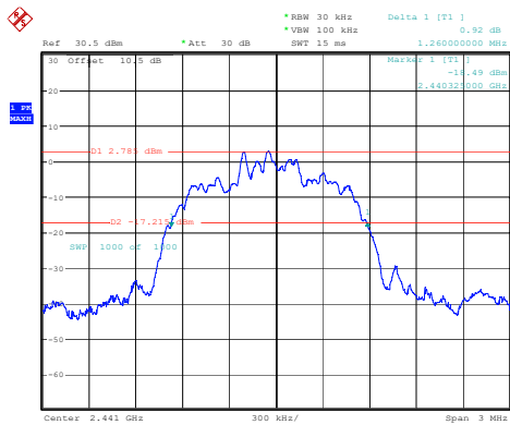
\pi/4 -DQPSK_Middle 1.260MHz
