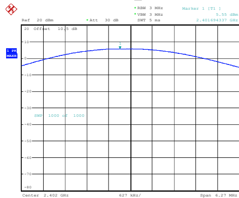
\pi/4 -DQPSK_Low 5.55dBm
