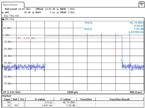
GFSK_Hopping_DH3 1.647ms
