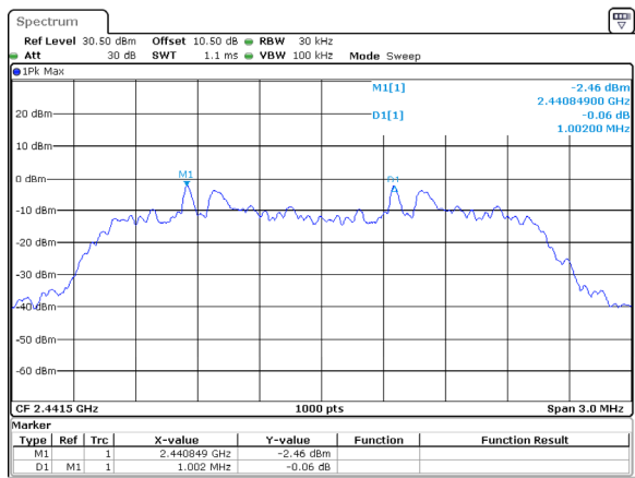
\pi/4 -DQPSK_Middle 1.002MHz
