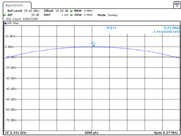
\pi/4 -DQPSK_Middle -0.01dBm
