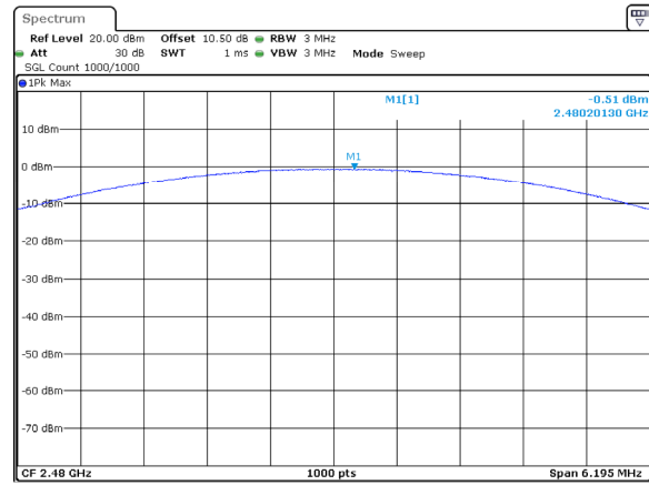
\pi/4 -DQPSK_High -0.51dBm
