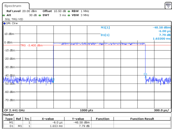
\pi/4 -DQPSK_Hopping_2DH3 1.653ms
