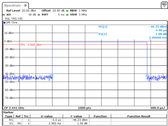
GFSK_Hopping_DH5 2.905ms
