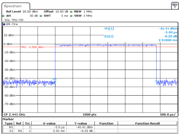
\pi/4 -DQPSK_Hopping_2DH5 2.910ms
