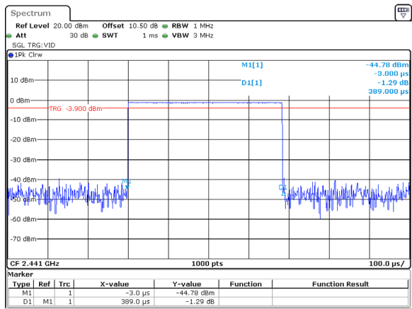
GFSK_Hopping_DH1 0.389ms
