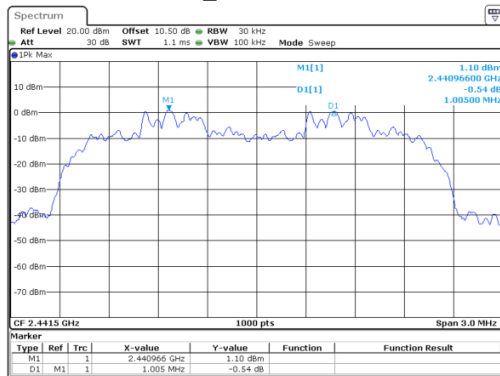
\pi/4 -DQPSK_Middle 1.005 MHz
