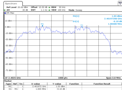
\pi/4 -DQPSK_Low 1.005 MHz
