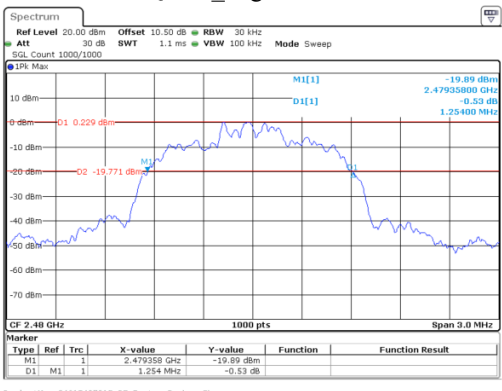
\pi/4 -DQPSK_High 1.254 MHz
