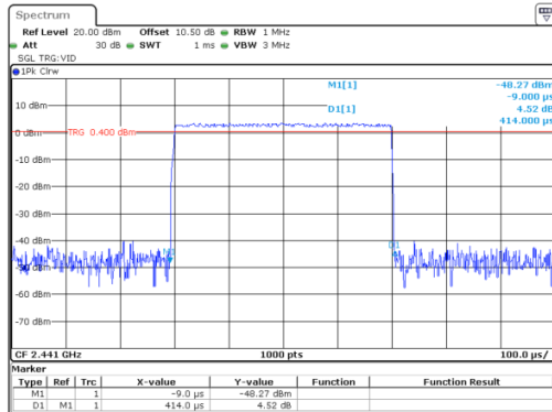
GFSK_Hopping_DH1 0.414ms
