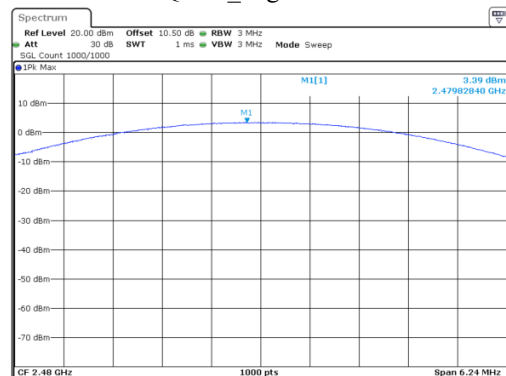
\pi/4 -DQPSK_High 3.39 dBm
