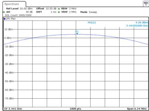
\pi/4 -DQPSK_Middle 4.26 dBm
