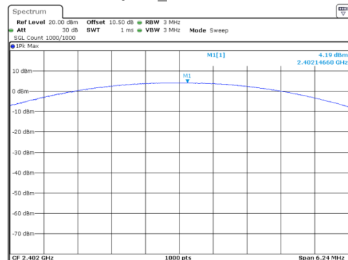
\pi/4 -DQPSK_Low 4.19 dBm
