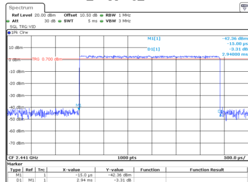
\pi/4 -DQPSK_Hopping_2DH5 2.940ms
