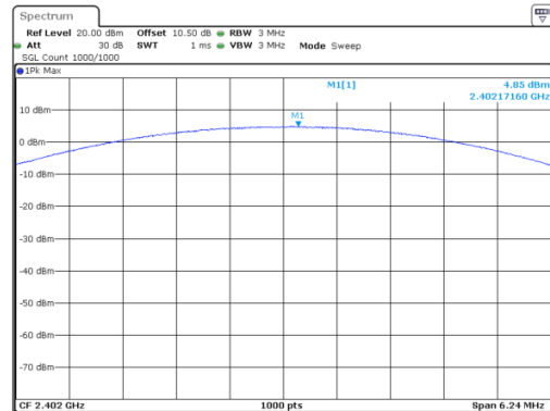
\pi/4 -DQPSK_Low 4.85 dBm
