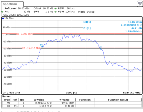
\pi/4 -DQPSK_Low 1.254 MHz
