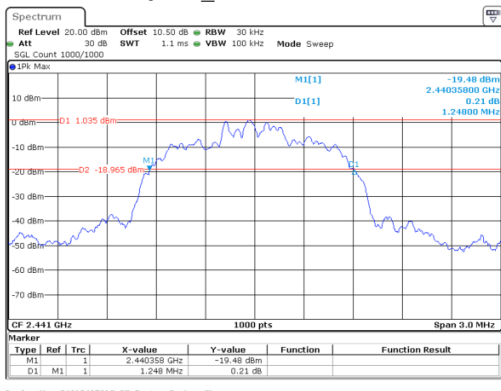
\pi/4 -DQPSK_Middle 1.248 MHz
