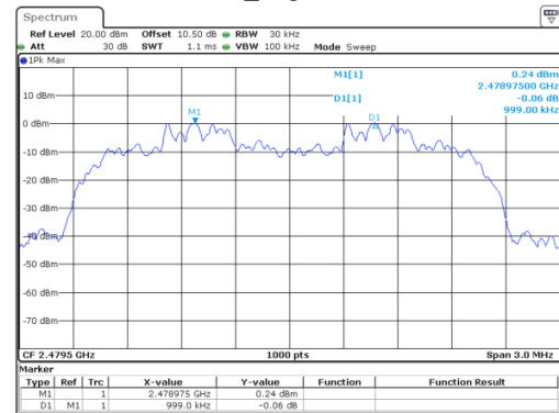
\pi/4 -DQPSK_High 0.999 MHz
