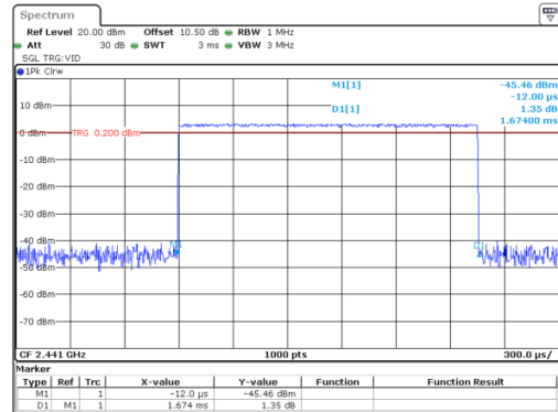
GFSK_Hopping_DH3 1.674ms
