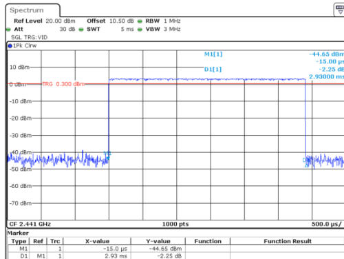
GFSK_Hopping_DH5 2.930ms
