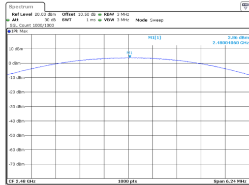
\pi/4 -DQPSK_High 3.86 dBm
