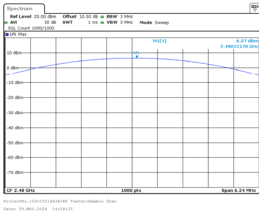
\pi/4 -DQPSK_High 6.57dBm
