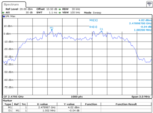
\pi/4 -DQPSK_High 1.002MHz
