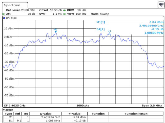
\pi/4 -DQPSK_Low 1.005MHz
