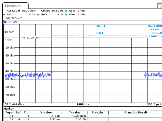
GFSK_Hopping_DH5 2.930ms
