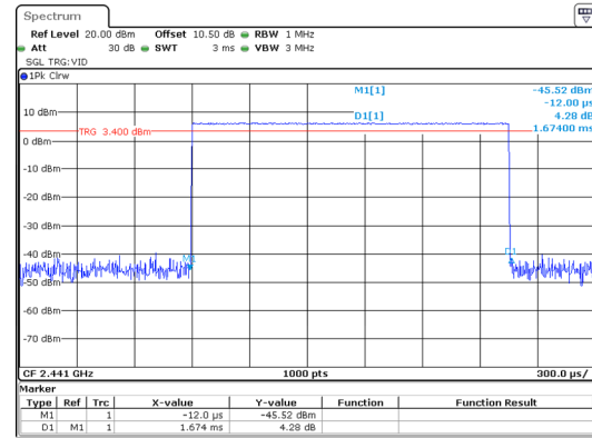
GFSK_Hopping_DH3 1.674ms
