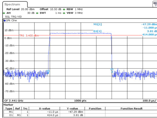
GFSK_Hopping_DH1 0.414ms
