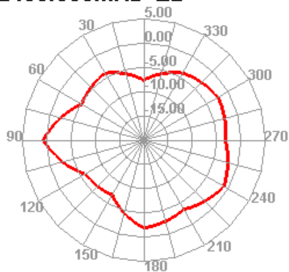
2450.000MHz E2
