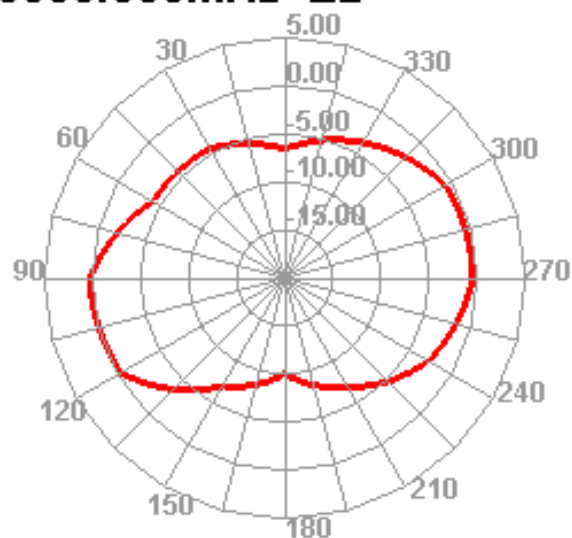
5500.000MHz E2
