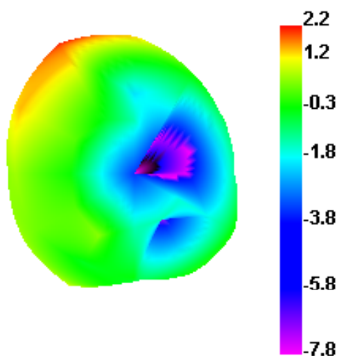
2450.000MHz
