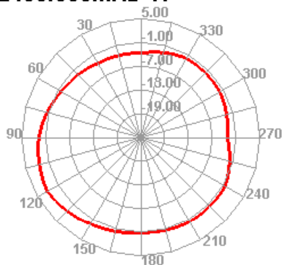
2450.000MHz H
