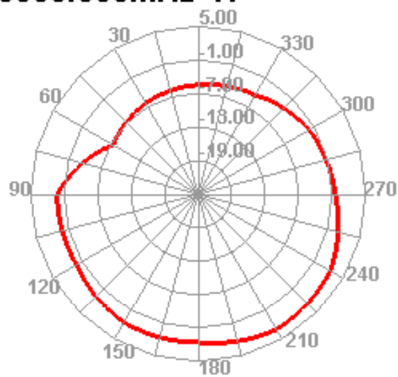
5500.000MHz H
