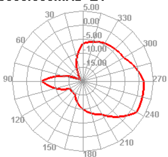
5500.000MHz E1
