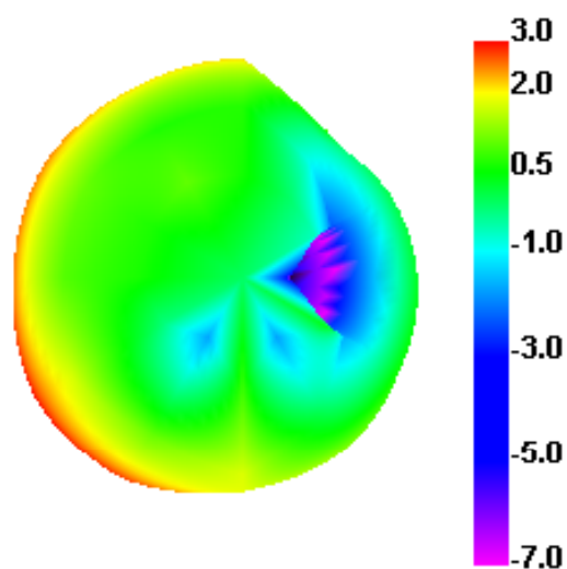
5500.000MHz E1
