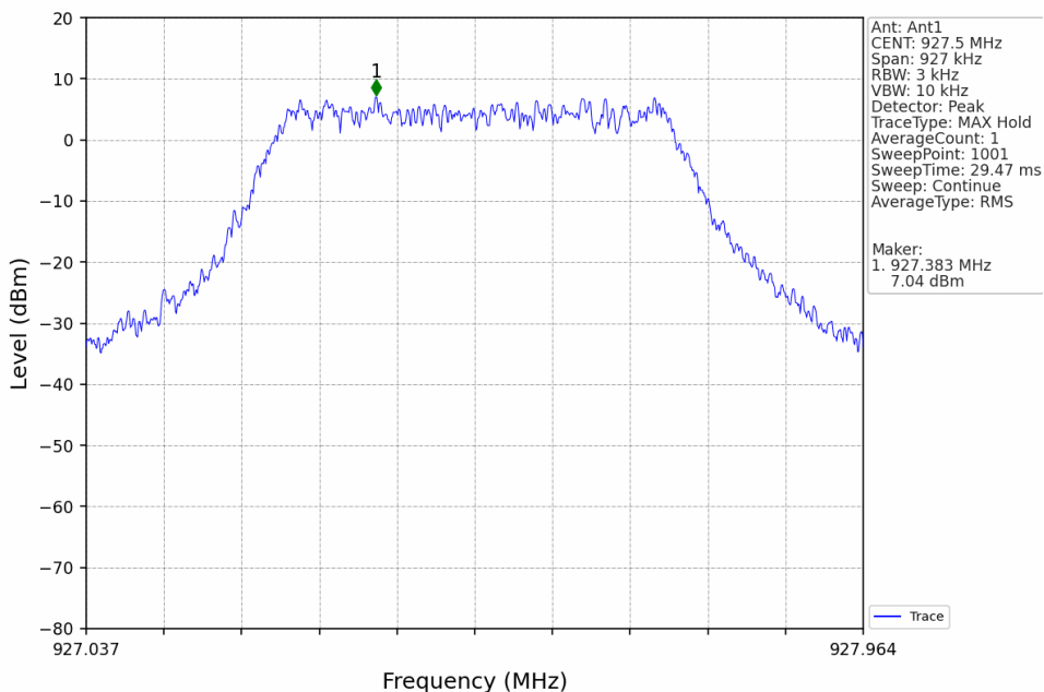
LORA_HCH_927.5MHz_Ant1_NTNV
