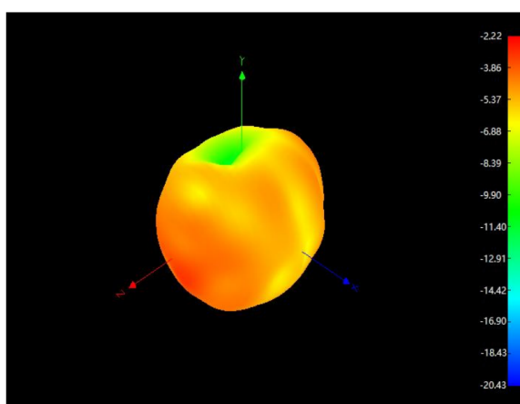
2480Mhz
