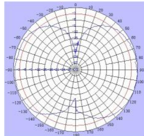
V 面方向图
