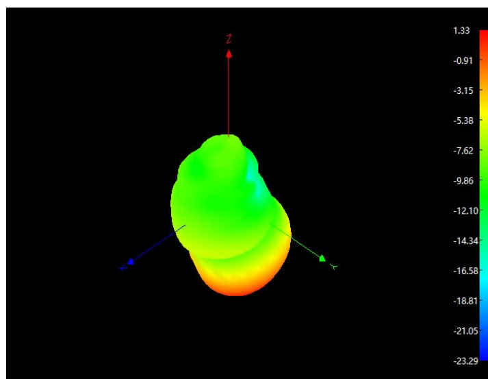
2500MHz 3D
