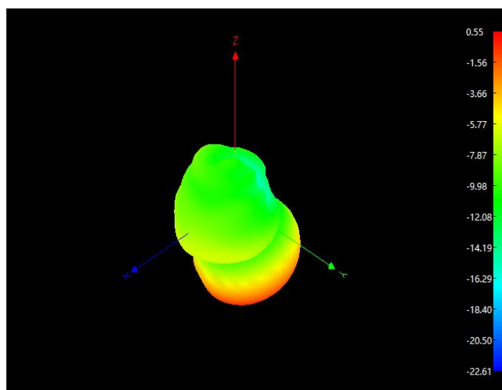
2450MHz 3D
