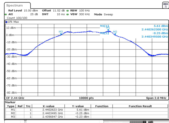
BLE 1M_Channel 19
