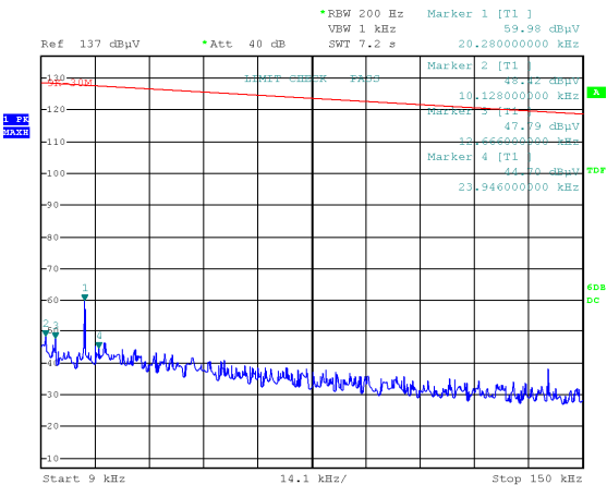
9kHz-150kHz
